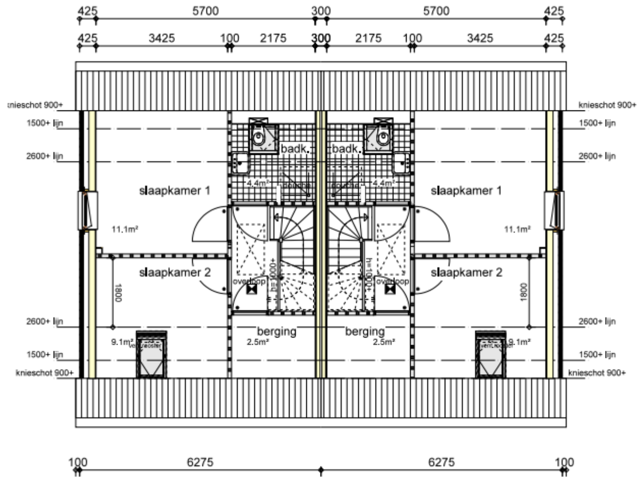
Verdieping 1 a 2 persoonswoning
