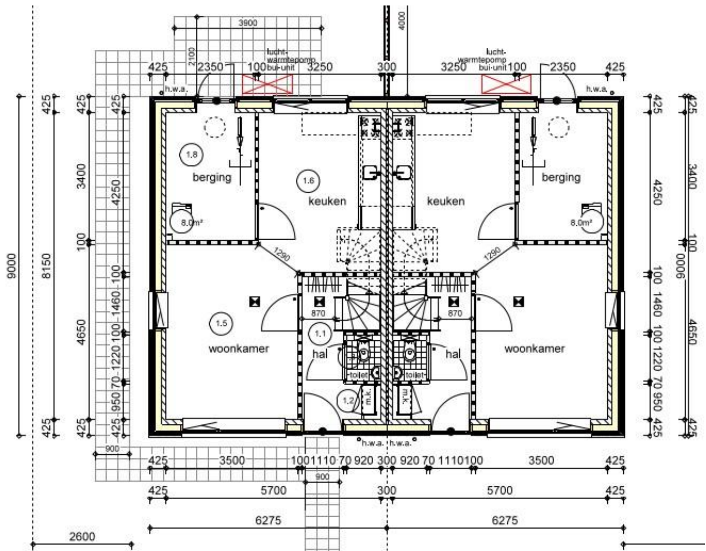
Begane grond 1 a 2 persoonswoning
