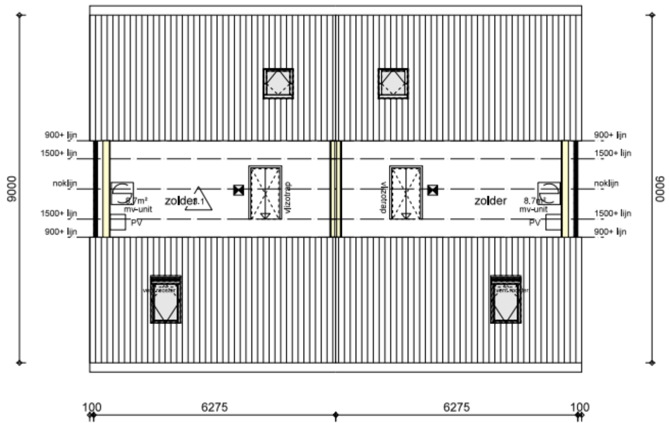
Zolder 1 a 2 woonswoning
